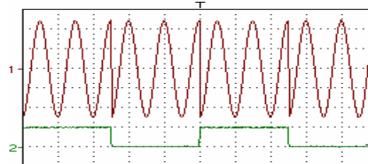
PSK INTERne : Voie1 : MAIN OUT Voie2 : VCG IN Sweep out
